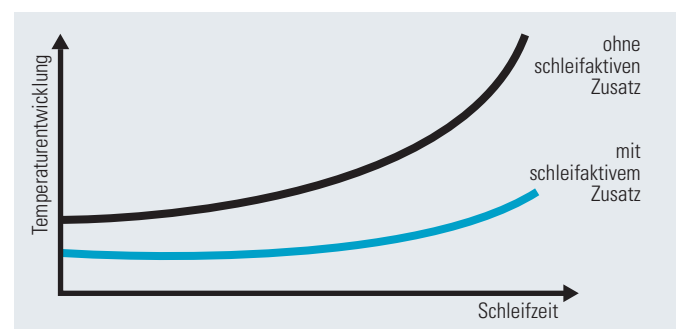
Kühler Schliff durch schleifaktive Zusätze
